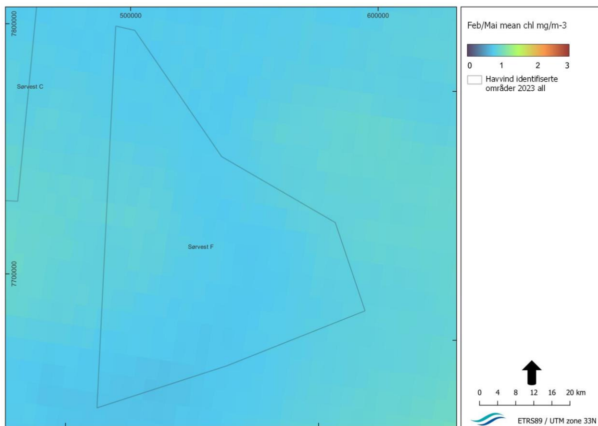
Figur 37 Gjennomsnitt av overflate klorofyll-a (i mg/m 3 ) for våroppblomstringsperioden (februar - mai) for de siste 20 år som indikator for planteplankton-produktivitet.
