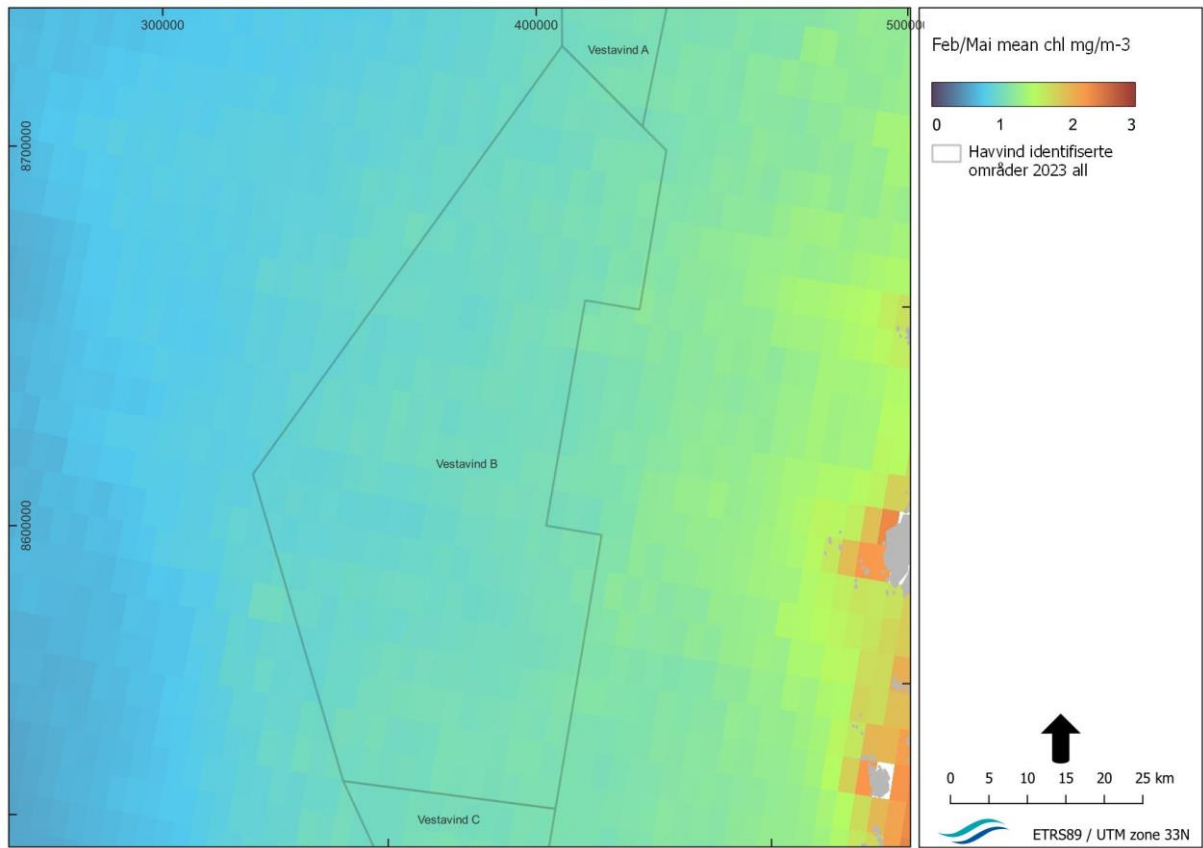
Figur 15 Gjennomsnitt av overflate-klorofyll-a (i mg/m³) for våroppblomstringsperioden (februar - mai) for de siste 20 år som indikator for planteplankton-produktivitet.
