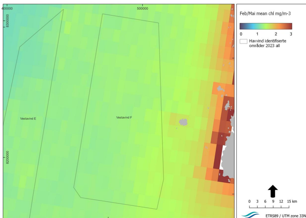
Figur 26 Gjennomsnitt av overflate-klorofyll-a (i \text{mg/m}^3 ) for våroppblomstringsperioden (februar - mai) for de siste 20 år som indikator for planteplankton-produktivitet.
