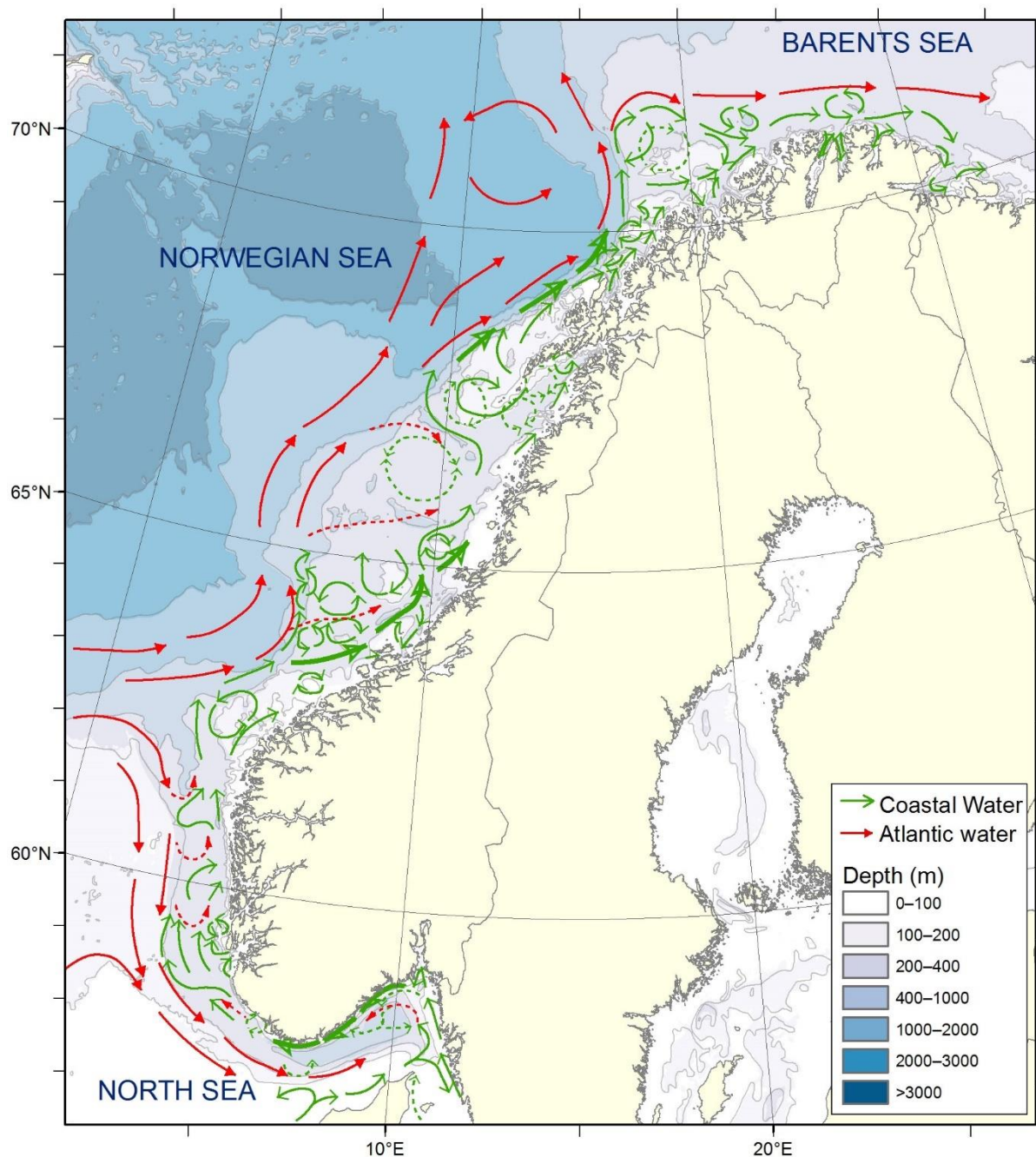
Figur 2 Kyststrømmen (grønne piler) har sin opprinnelse i Østersjøen og er sterkest langs kysten. Atlantisk vann med opprinnelse i Mexicogulfen strømmer langs sokkelkanten utenfor kyststrømmen (røde piler). Figur fra Havforskningsinstituttet (2020).
